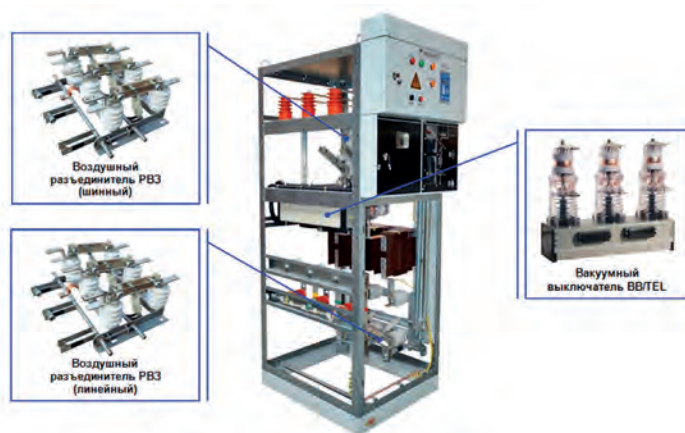
КСО-207 «Оскол» с двумя воздушными разъединителями
