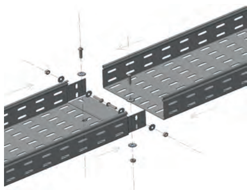
Монтаж ЛМс-П3М "без соединителя"
