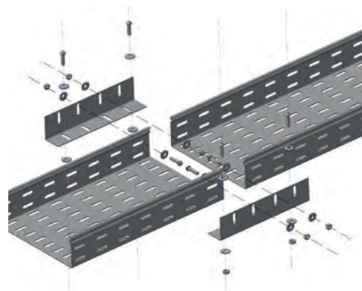
Монтаж ЛМс-П3 с помощью соединителя
